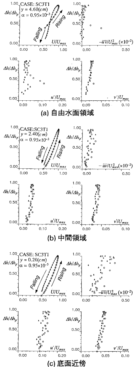
図-6 水深変化 \Delta h に対する平均流速 U 、乱れ強度 u'v' およびReynolds応力 -\overline{uv} の変化
