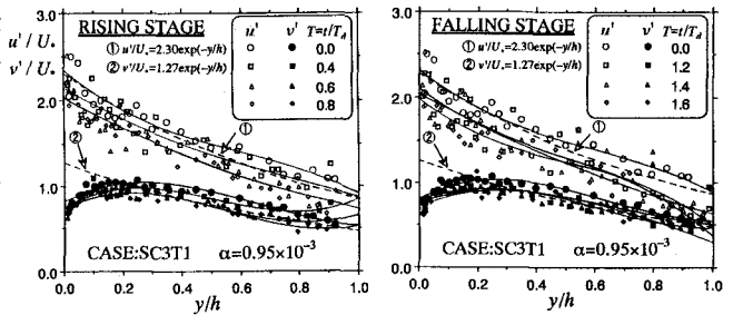
図-1 乱れ強度分布
