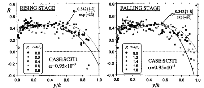
図-3 相関係数
