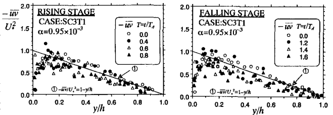
図-2 Reynolds応力分布
