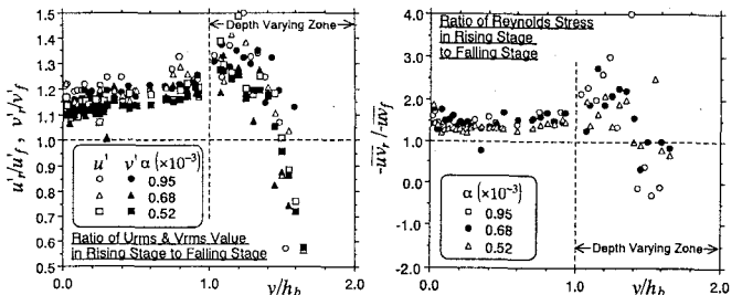
図-4 乱れ強度の平均値の比 図-5 Reynolds応力の平均値の比
