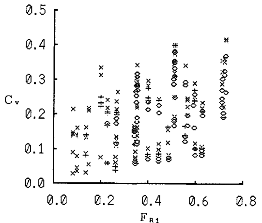
図-4 閉塞限界(45度屈曲部)
