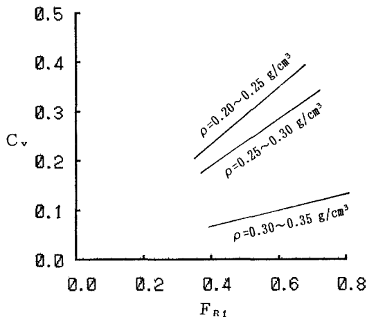
図-5 閉塞限界(90度屈曲部)
