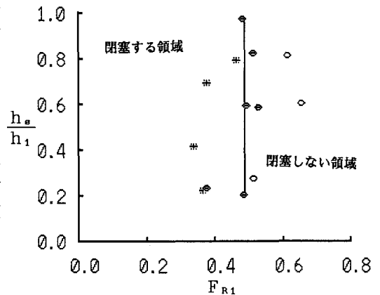
図-2 閉塞限界(90度屈曲部)
