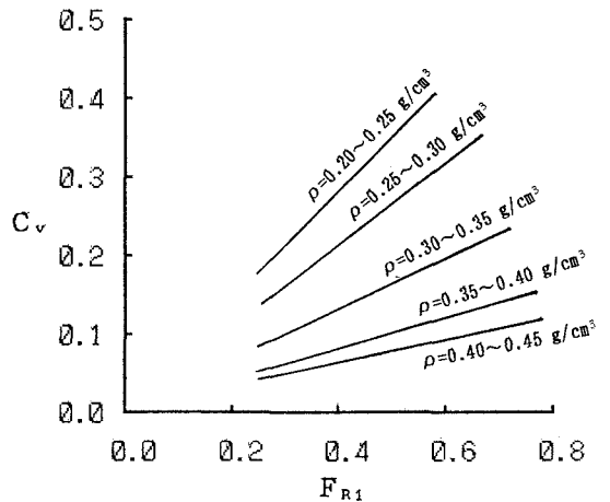
図-6 閉塞限界(45度屈曲部)
