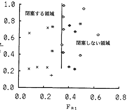
図-3 閉塞限界(45度屈曲部)
