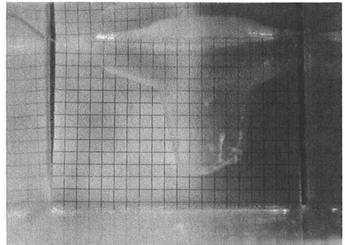
b)NaI水溶液中( n=1.406 )
