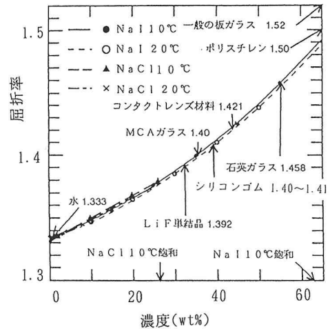
図-1 屈折率と濃度の関係
