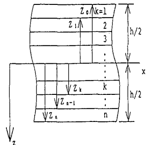
図-1 一般図
