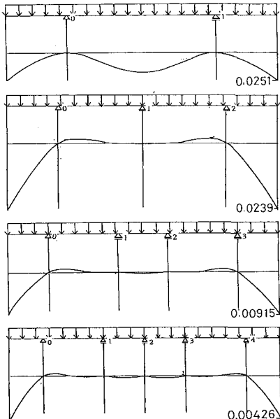
図-5 支点位置と変形
