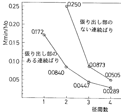
図-3 径間数と最小曲げモーメント
