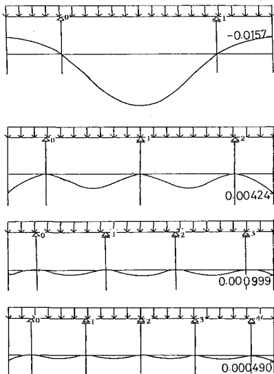
図-4 支点位置と変形
