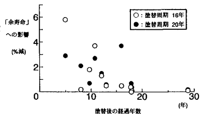
図-5 台風が余寿命に及ぼす影響
