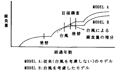
図-2 台風の影響を考慮した
