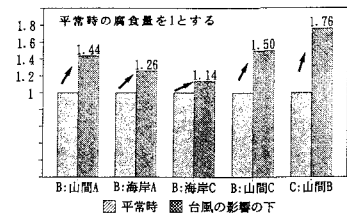
図-4 台風が鋼材腐食に及ぼす影響
