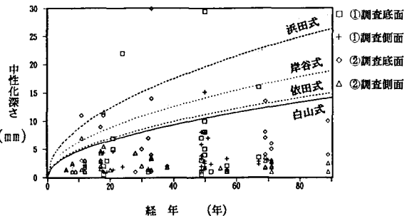
図-2 経年と中性化深さ
