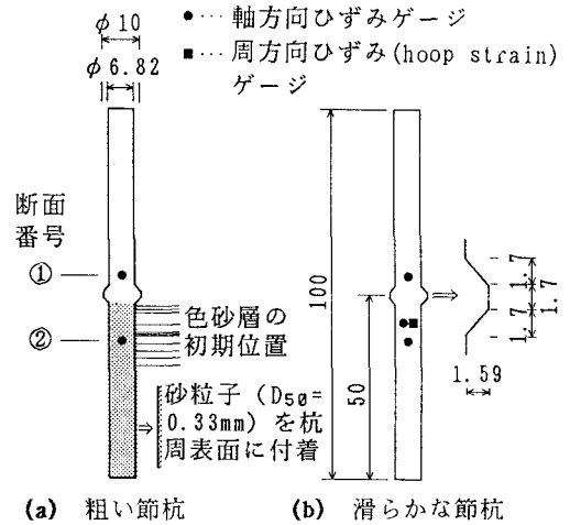
図-1 モデル節杭（単位：cm）
