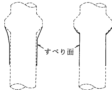
(a) 粗い節杭 (b) 滑らかな節杭
