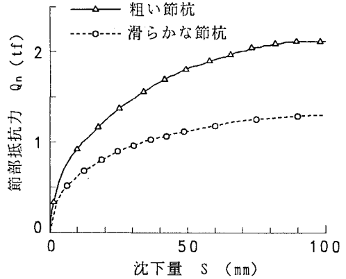
図-2 節部抵抗力-沈下量関係
