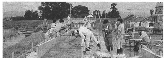
写真1 植生層上流れの現地実験（梯川）
