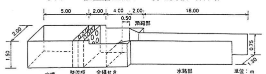
図1 実験水路
