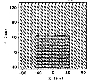
図1 50m高度における初期風速の水平分布
