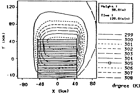
図3 50m高度における温位の水平分布
