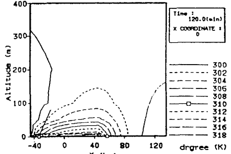
図4 鉛直断面内の温位分布
