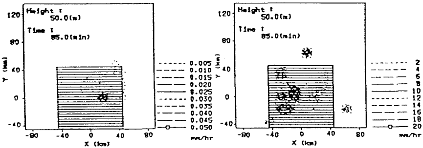
図5 85分後の暖かい雨(左)と対流による雨(右)の降雨強度分布
