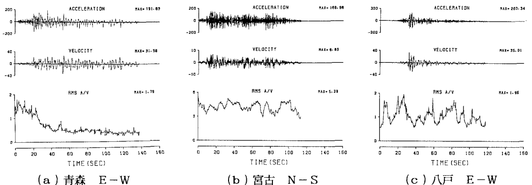
図-1 加速度および速度の時刻歴と a_{rms}(t)/v_{rms}(t)/2\pi の時間的変動
