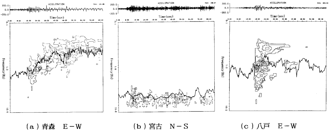
図-2 rms 振幅比 a_{rms}(t)/v_{rms}(t)/2\pi と非定常パワースペクトル
