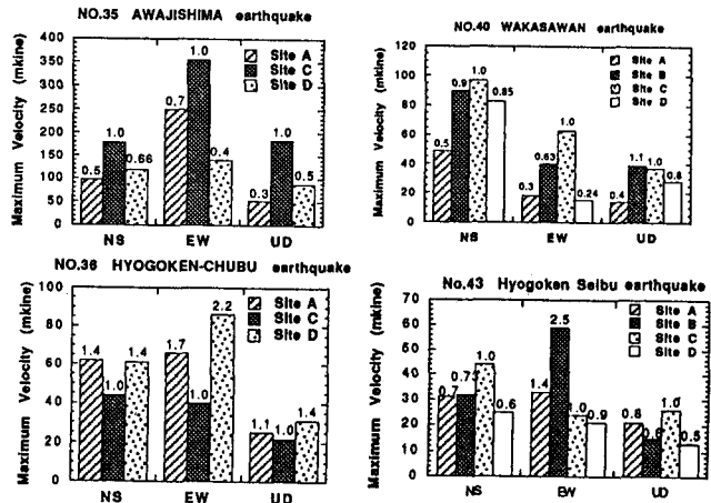
Fig-6 最大速度比 ( / C)
