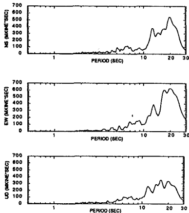
Fig-3 フーリエスペクトル (No.38: 明石市)
