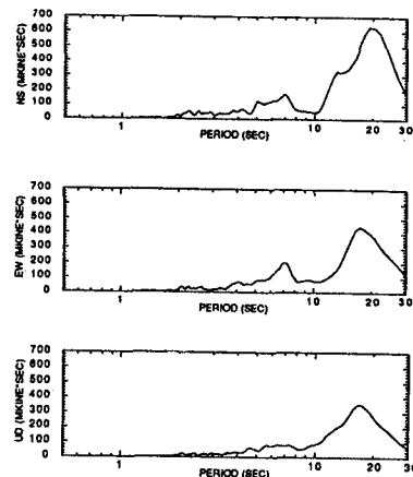
Fig-4 フーリエスペクトル (No.38: 淡路島)
