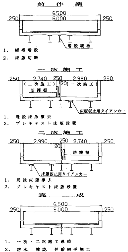
図-4 施工要領
