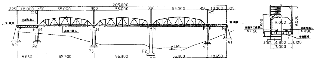
図 - 1 一 般 図
