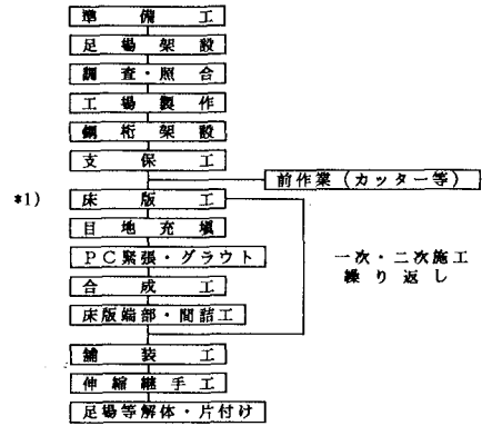
図-3 施工のフローチャート
