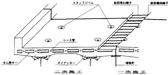
図-2 プレキャスト床版の構造
