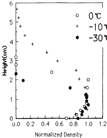
図-2 a 温度による変化
