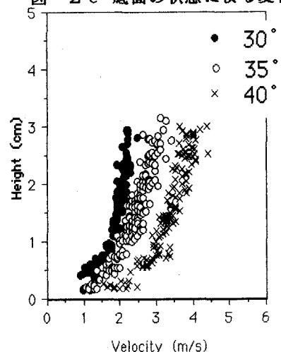
図-3 b 傾斜角による変化
