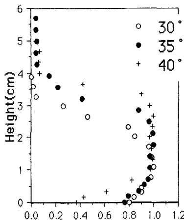
図-2 b 傾斜角による変化
