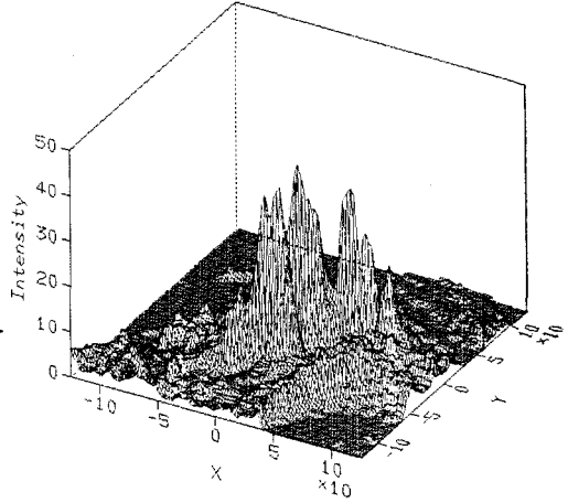
図6 実際の降雨場
