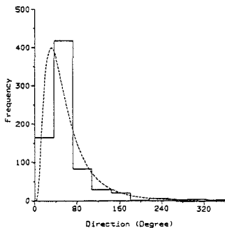
図2 移動方向の分布図
