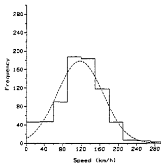
図3 速さの分布図
