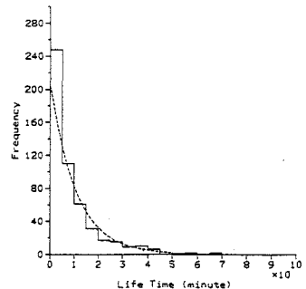
図4 寿命の分布図
