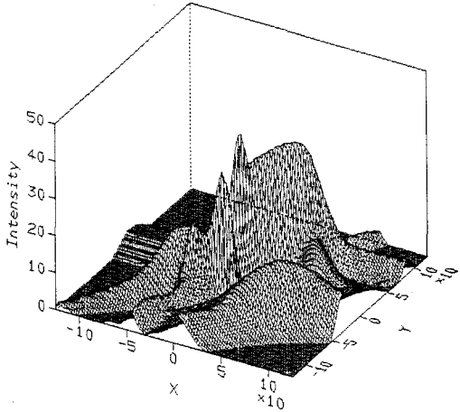
図5 近似した降雨場
