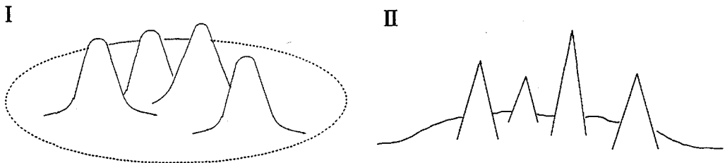
図7 降雨場のモデル化
