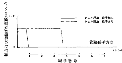
図.9 軸方向の地盤ばね定数
