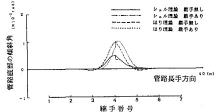
図.8 管路頂部の傾斜角
