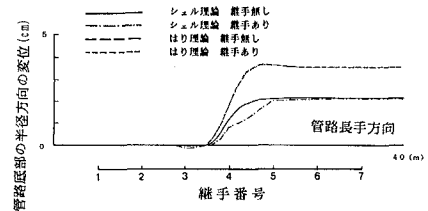
図.7 管路底部の半径方向変位
