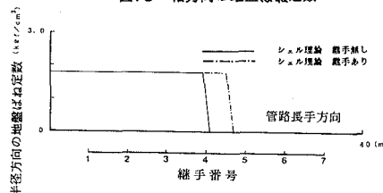
図.10 半径方向の地盤ばね定数
