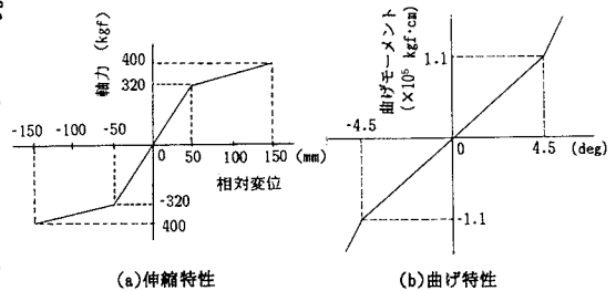
図.3 ジョイント特性
