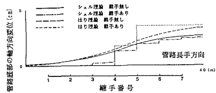
図.6 管路底部の軸方向変位
