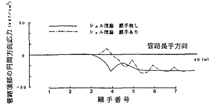
図.5 管路頂部の円周方向応力の分布
