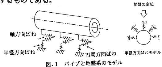
図.1 パイプと地盤系のモデル
