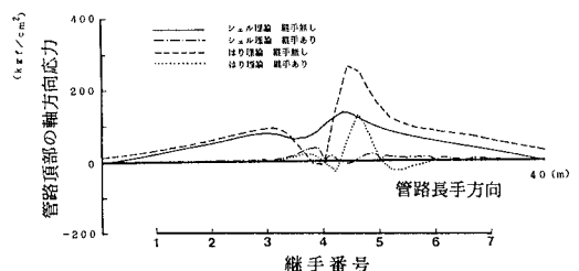
図.4 管路頂部の軸方向応力の分布
