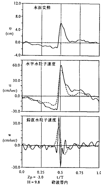
図2 巻き波型砕波 (CASE - 2)
