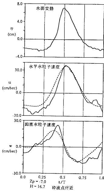
図1 崩れ波型砕波 (CASE - 1)
