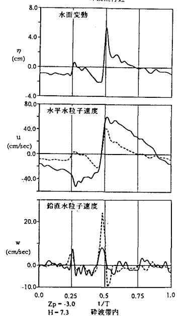
図3 砕け寄せ波型砕波 (CASE - 3)
