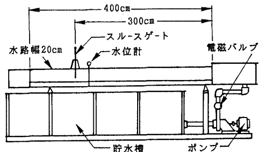
図-1 循環式開水路実験装置
