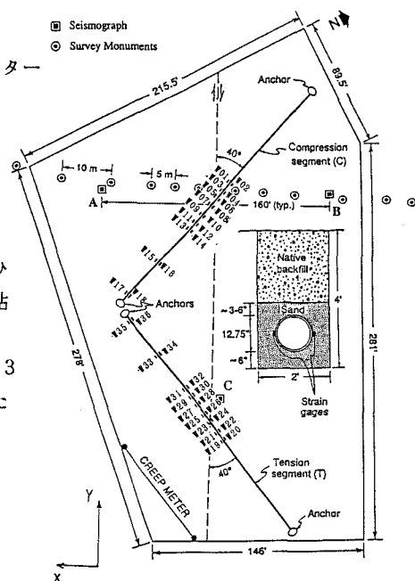
図1 Parkfield 観測システム
