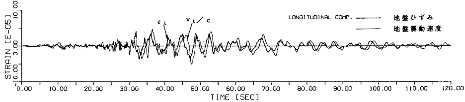
図4 地盤ひずみと地盤の震動速度の比較
