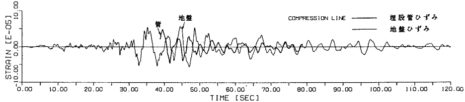
図5 地盤ひずみと埋設管ひずみの比較
