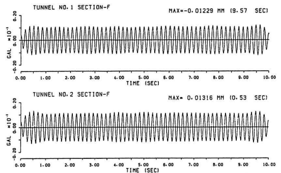
図-4 継手部相対変位波形（N0.1；免震構造）
