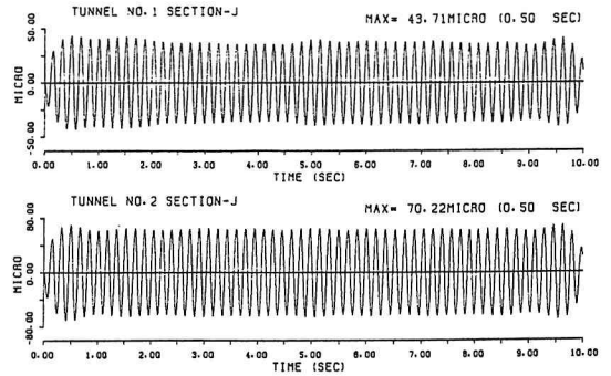
図-3 トンネルひずみ波形（N0.1；免震構造）
