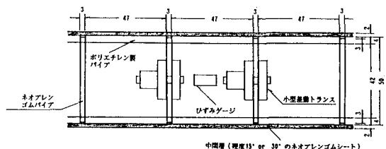
図-2 トンネル模型の縦断面図
