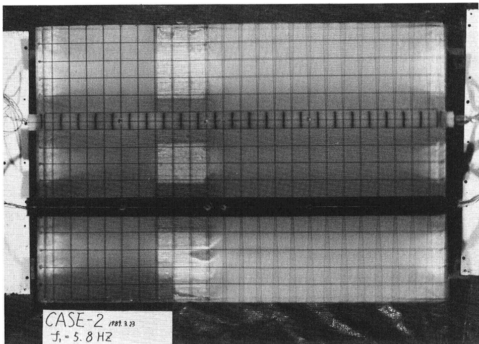
写真-1 模型振動実験ブレ写真（CASE-2）
