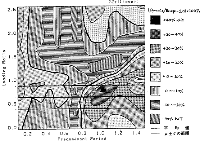
図3 バンド幅0.1の極めて狭帯域の地震動入力に対する大型車の積載率と地震応答の関係（橋梁下端曲げモーメント）
