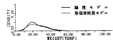
(8) 全重量に関する周辺分布
