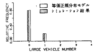
(4) 大型車の台数を条件とする全重量の条件付分布
