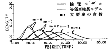
(6) 大型車の台数を条件とする全重量の条件付分布
