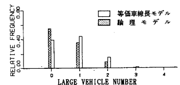
(7) 大型車の台数に関する周辺分布
