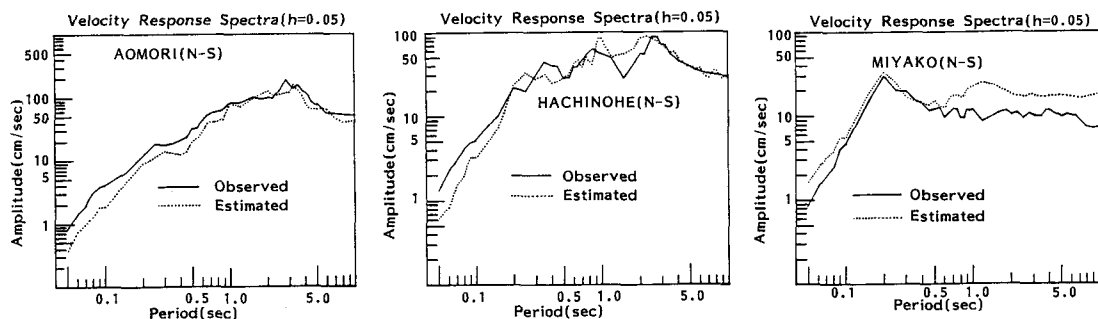
図5 (2) 改良震源モデルによる応答スペクトルの比較
