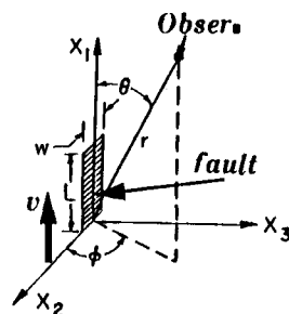
図2 一樣断層モデル
