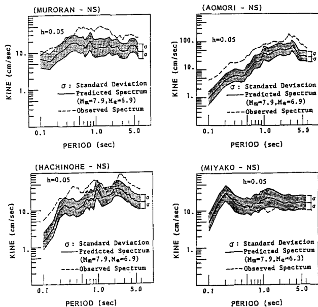
図4 点震源モデルによる応答スペクトルの比較
