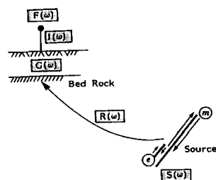
図1 地盤震動の模式図
