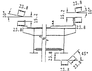
図-6 制振装置付設断面図
