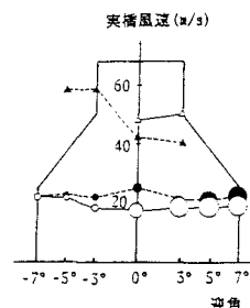
図-8 V_{cr} - \alpha 曲線 （断面C）
