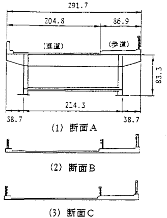
図-1 橋桁断面図
