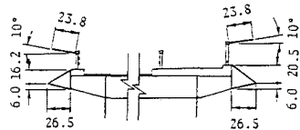
図-9 制振装置付設断面図 （Fairing + One flap）
