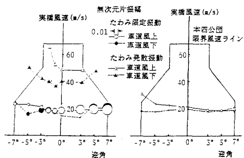
図-5 V_{cr} - \alpha 曲線 （断面B）
