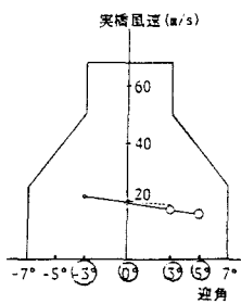
図-10 V_{cr} - \alpha 曲線 （断面C + 制振装置）
