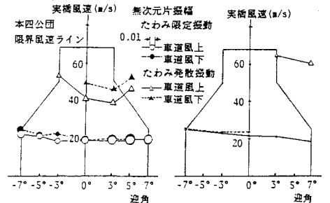
図-2 V_{or}-\alpha 曲線 (断面A)
