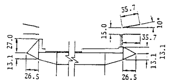
図-3 制振装置付設断面図 (Double flap + Fairing)
