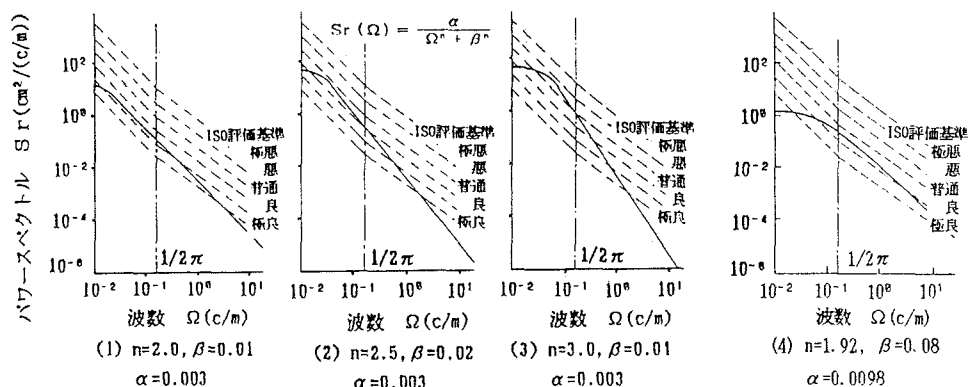
図-3 路面凹凸スペクトル
