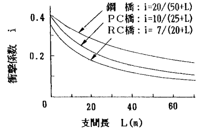
図-1 衝撃係数
