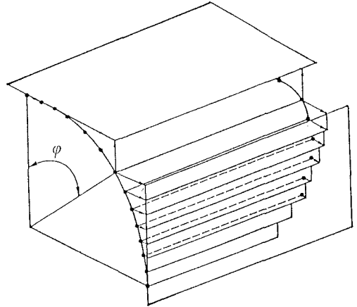
Fig. 4 コーナー部を投影したモデル
