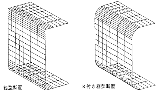
Fig.3 要素分割
