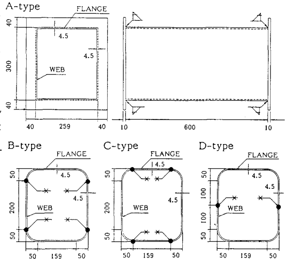
Fig.1 供試体 (unit:mm)
