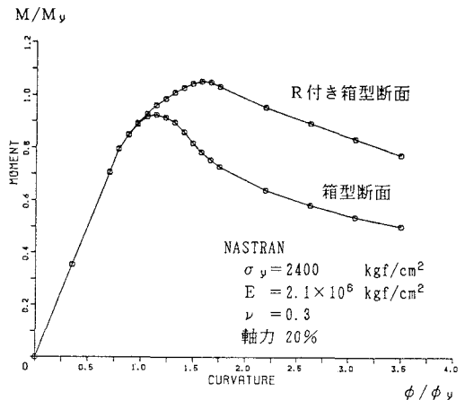
Fig. 5 NASTRAN による解析結果
