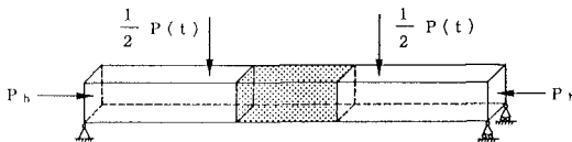
Fig.2 载荷形式
