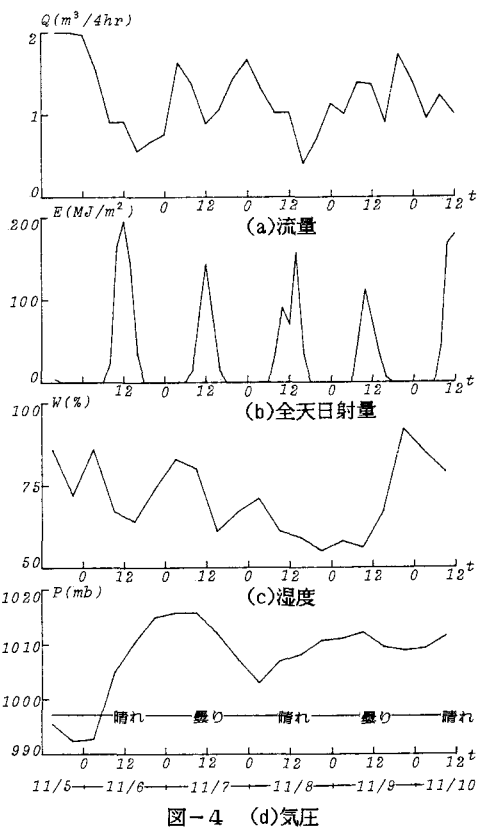
図-4 (d)気圧
