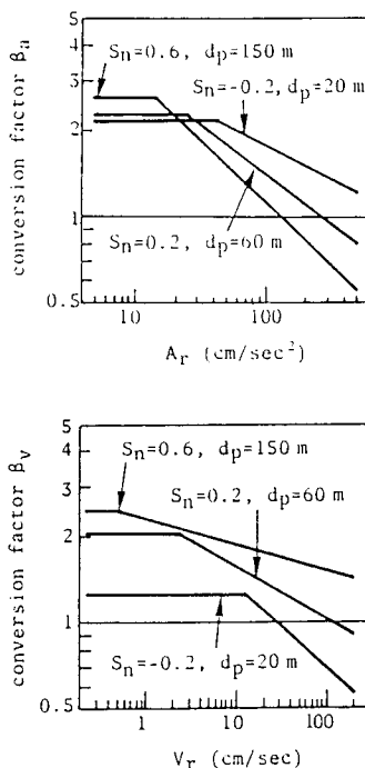
図-1 種々の S_n \cdot d_p による \beta の推定値
