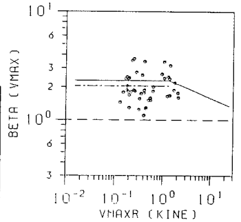
図-2 地震動の増幅率と地震動変換係数の関係
