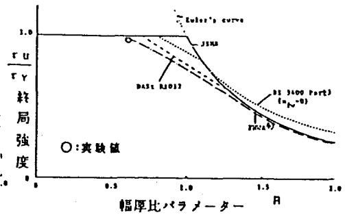
図-3(b) 終局強度曲線( \tau_u/\tau_y )
