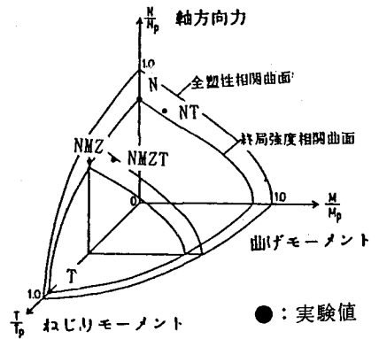
図-4 強軸曲げが作用したときの終局強度曲面
