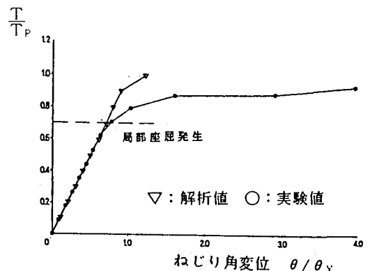
図-2 ねじりモーメント・ねじり角曲線(T-1)
