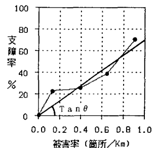
図1 支障率と被害率の関係を示す特性値（回帰直線の傾き： \tan \theta ）
