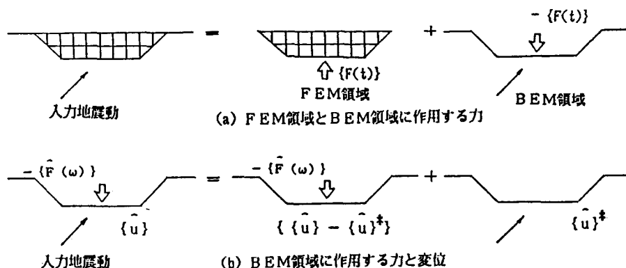
Fig-2.1 FEM領域とBEM領域に作用する力と変位
