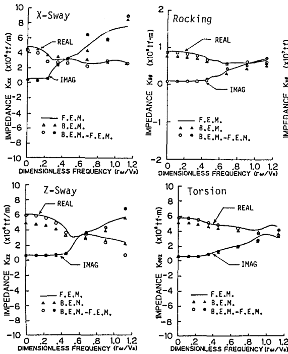
図3 ケーソン重心におけるインピーダンス関数
