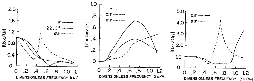
図6 有効入力動（ケース2）
