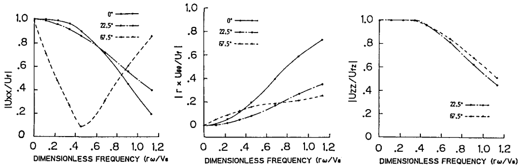
図5 有効入力動（ケース1）
