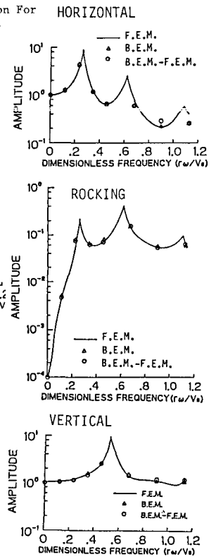
図4 ケーソン重心における振動数応答
