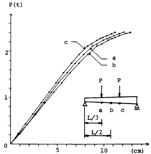
図-4 荷重-変位曲線 (No.10)
