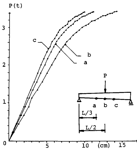
図-3 荷重-変位曲線 (No.3)
