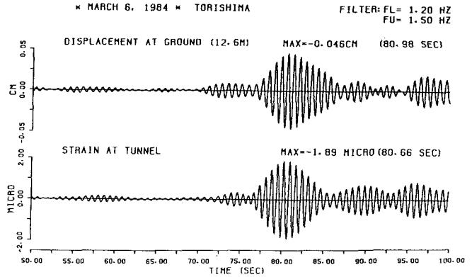
図-3 地盤変位と洞道軸ひずみの比較図(鳥島近海地震)
