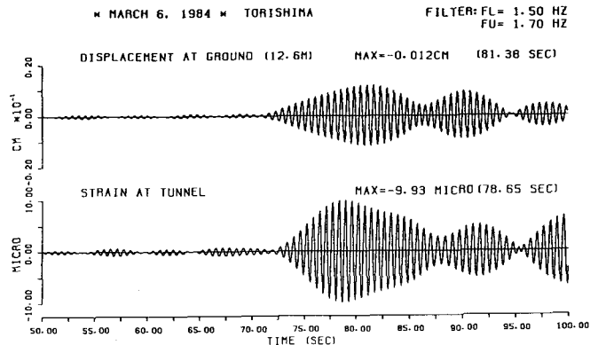
図-5 地盤変位と洞道軸ひずみの比較図(鳥島近海地震)
