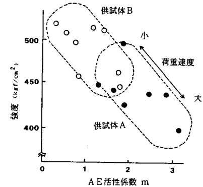
図-5 強度 \sim m 関係
