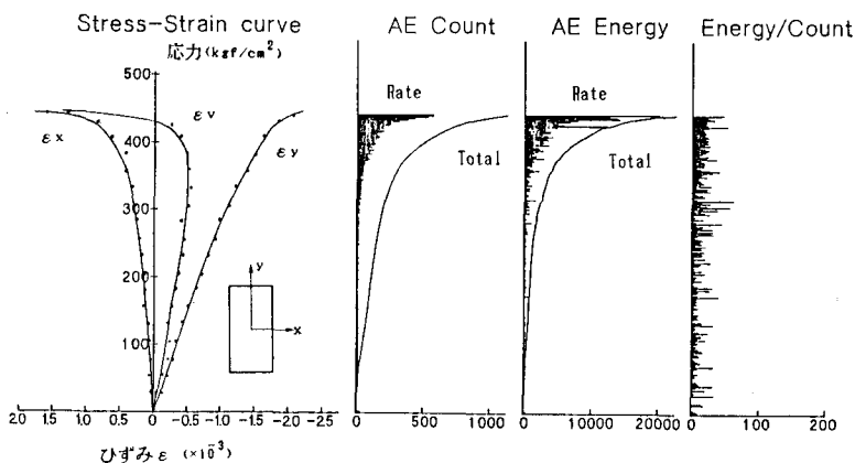
図-2 \sigma \sim \varepsilon とAE特性
