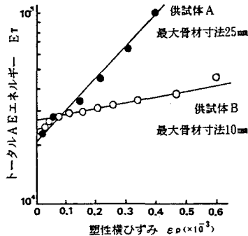
図-3 E_T \sim \varepsilon_p 関係
