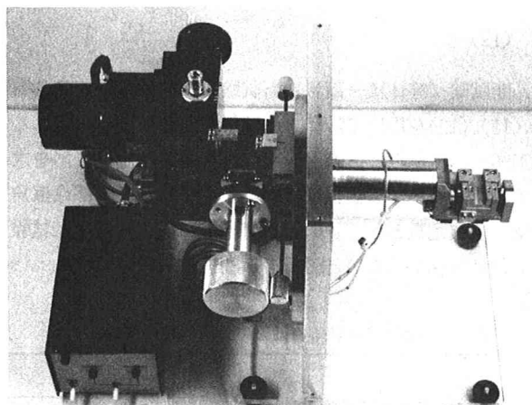
写真-1 超小型せん断試験機
