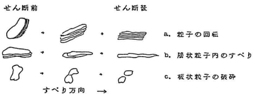
図-3 せん断によるベッドの変形
