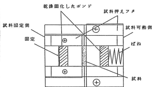
図-1 試料ホルダー部
