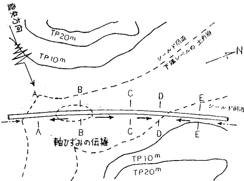
図-4. 軸ひずみの伝播模式図
