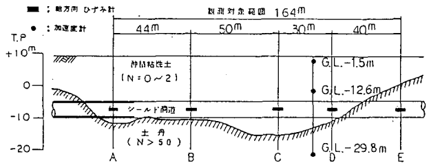
図-1. 縦断面図
