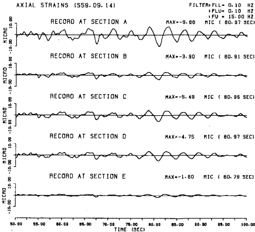
図-3. 軸ひずみ記録
