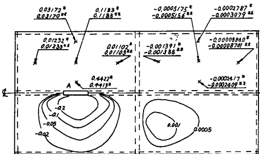
換算せん断力 ( V_x ) の影響面 (A点)
