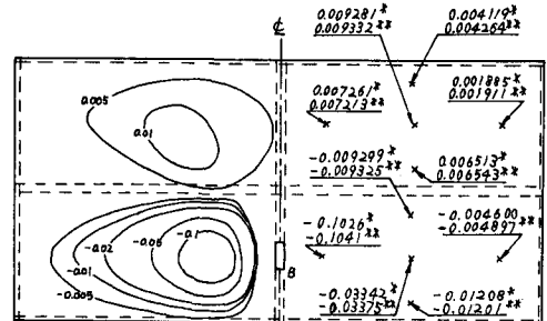
曲げモーメント ( M_x ) の影響面 (B点)
