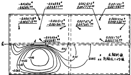
曲げモーメント ( M_x ) の影響面 (A点)
