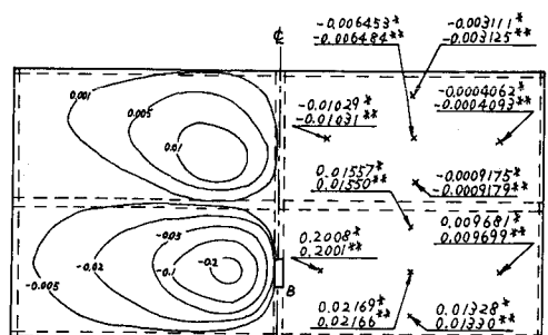
換算せん断力 ( V_x ) の影響面 (B点)
