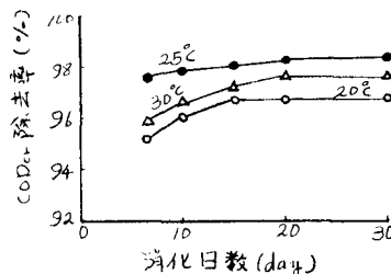
図2. \text{COD}_{\text{Cr}} 除去率と消化日数
