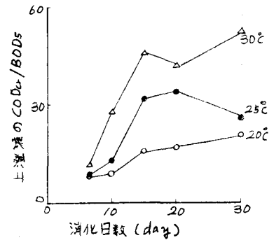
図4. 上澄液の COD_{Cr}/BOD_5 と消化日数
