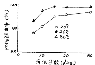
図3. BOD 5 除去率と消化日数
