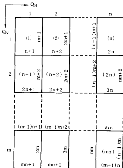
図-3 メッシュ型管網
