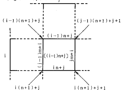
図-4 i 行 j 列の部材番号
