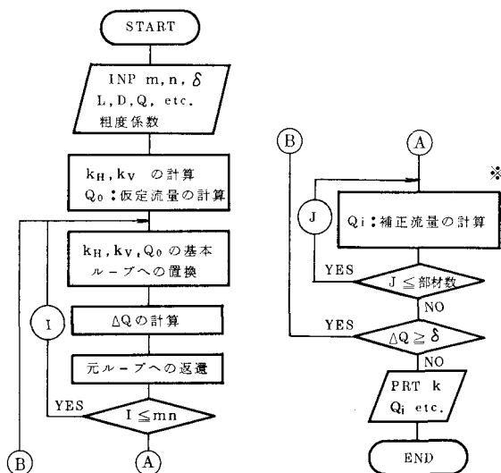
図-7 メッシュ型管網のフロー図
