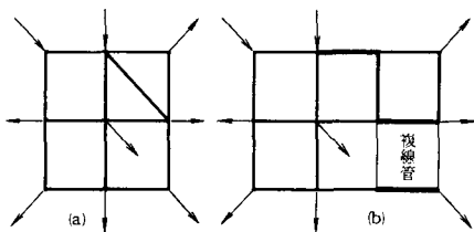
図-2 等価管網の例
