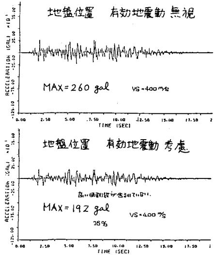
図-4 地盤位置での応答加速度波
