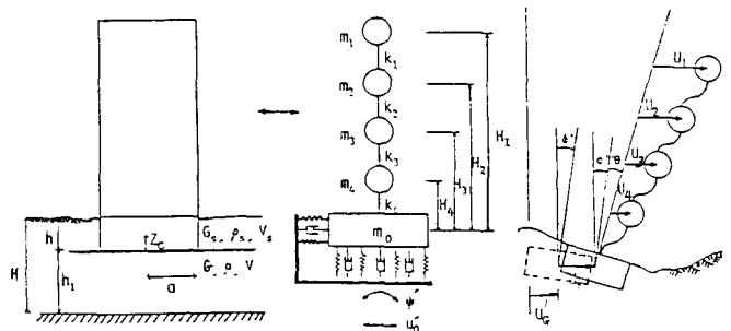
図-1 地盤-構造物モデルとその記号
