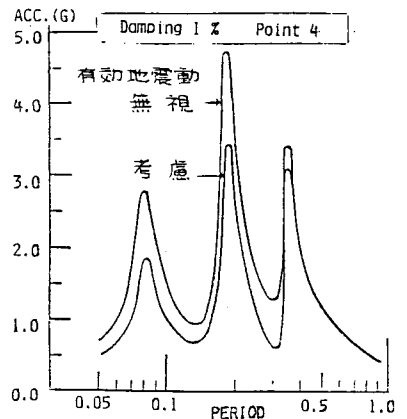
図-6 質点4の応答スペクトル
