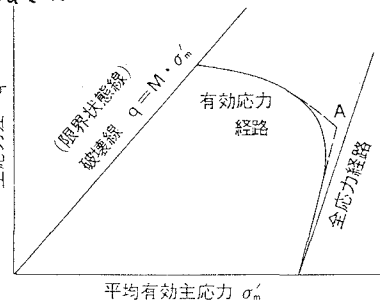
図-2 非排水三軸圧縮試験の応力経路
