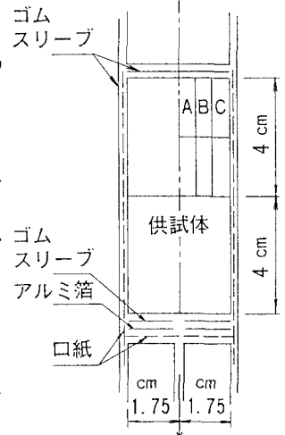
図-1 三軸試験供試体
