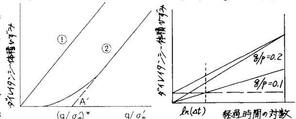
図-3 ダイレイタンシーが生じる応力比
