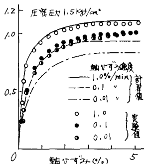
図-5 定Vで速度試験主応力差
