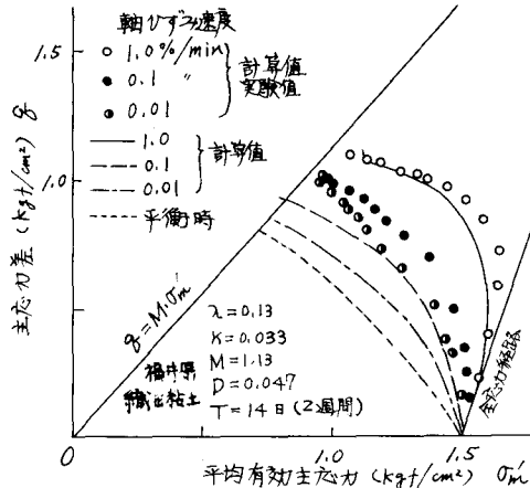
図-11 定Vで速度試験主応力差
