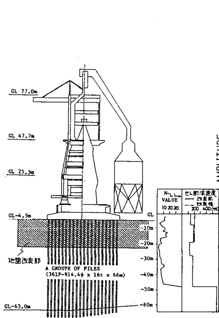
図2.大型高炉
