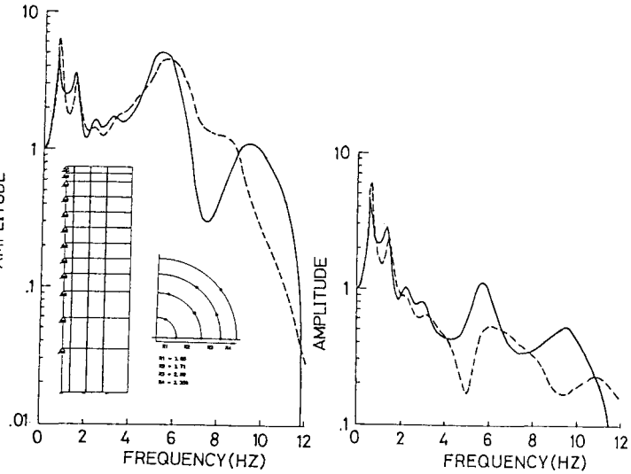
図3.振動数応答関数（橋脚）
