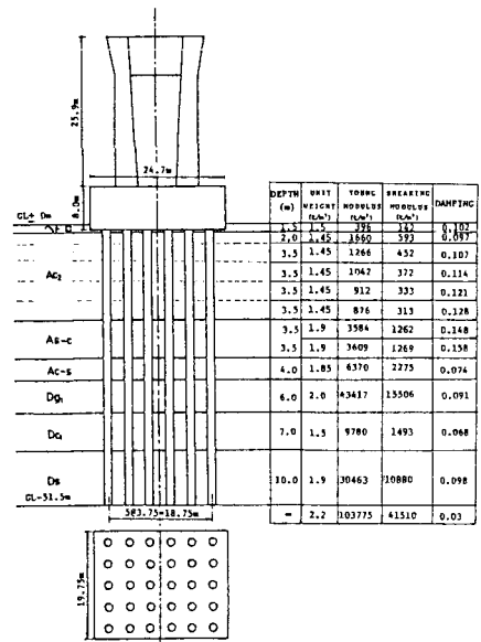
図1.橋脚
