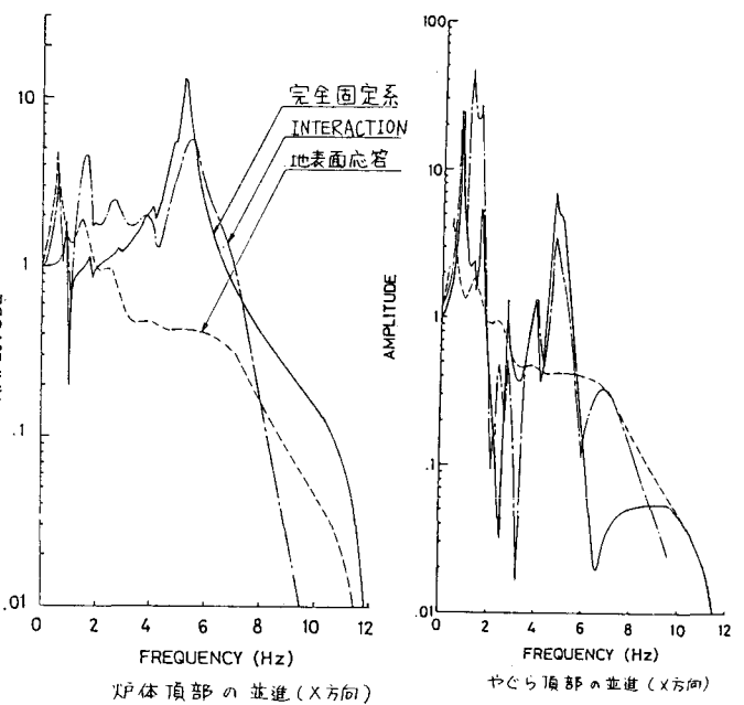
図4.振動数応答関数（高炉）
