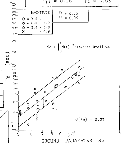
図-3 S_c と卓越周期 T_g の関係 (データ数 29)
