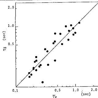
図-4 予測値 \bar{T}_g と実測値 T_g の関係
