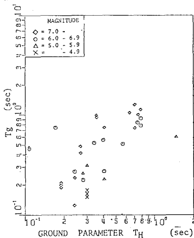
図-1 T_H と卓越周期 T_g の関係
