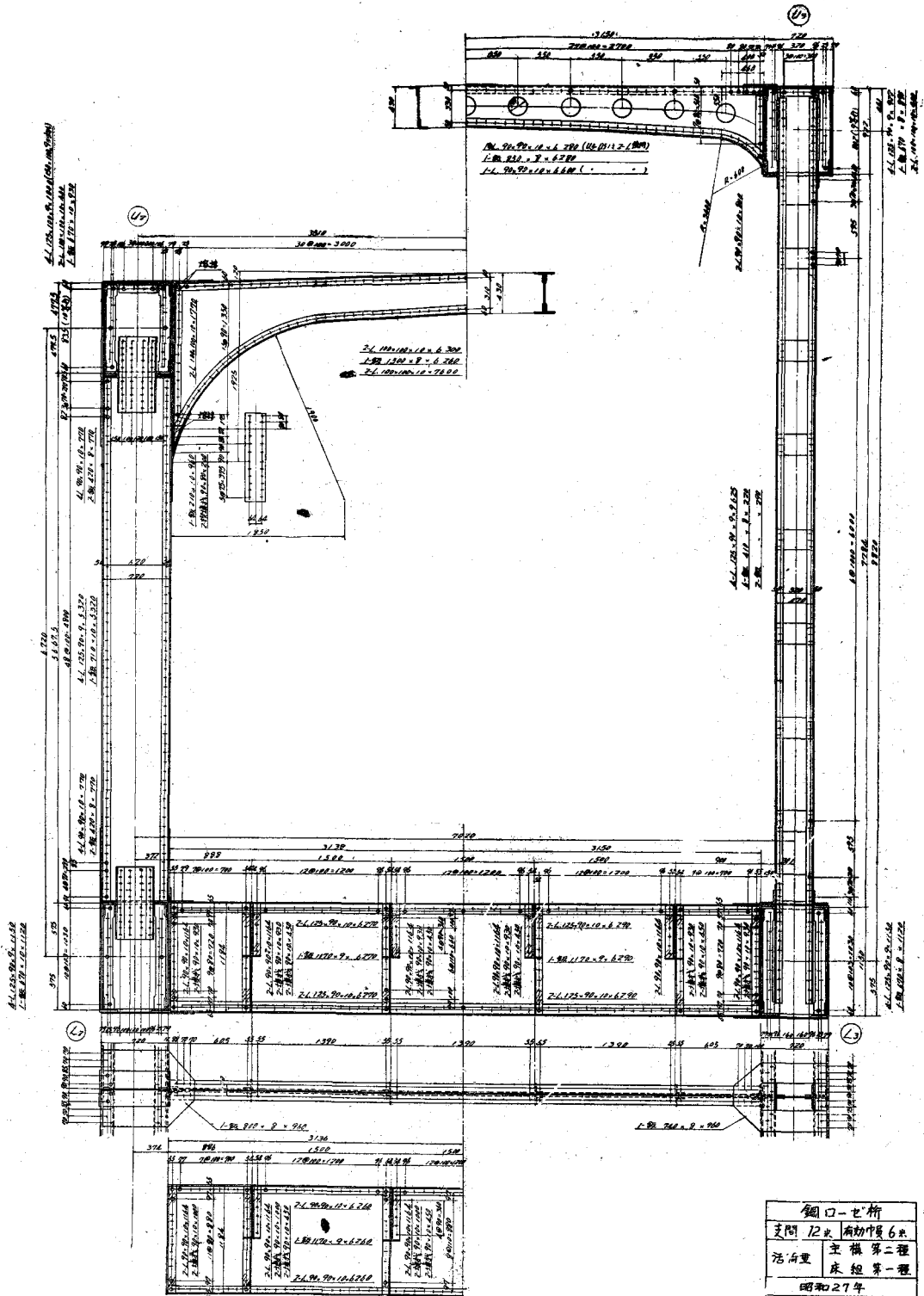
図-3 鋼口一セ桁橋門構詳細図
