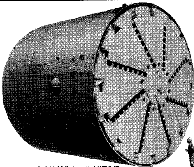
●6.99mφ 完全機械化シールド掘進機
