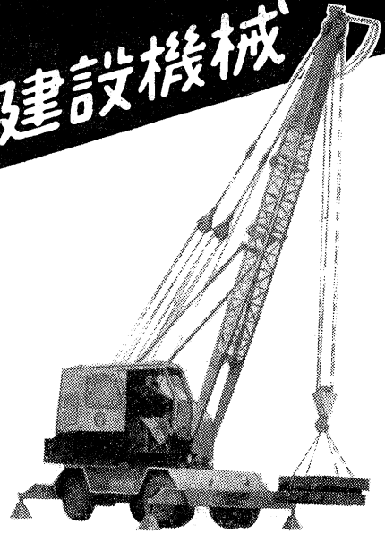
205型 クルーザークレーン 吊上重量 12.7 屯 走行速度 13km/h
