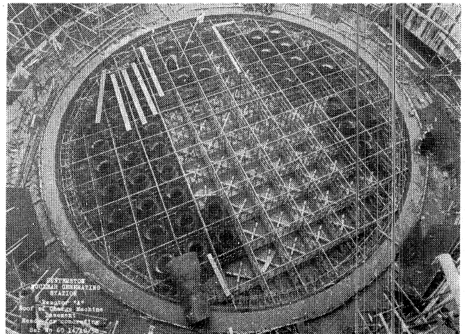
Hunterston 原子炉Aの基礎 Charge Machine（燃料装脱機）の Sleeve（円筒形のもの）のコンクリート打設直前の状況。この Sleeve を通して燃料を出入する。この真上に原子炉圧力容器をすえつける。ごぼん目に見えるのは鉄筋である。
