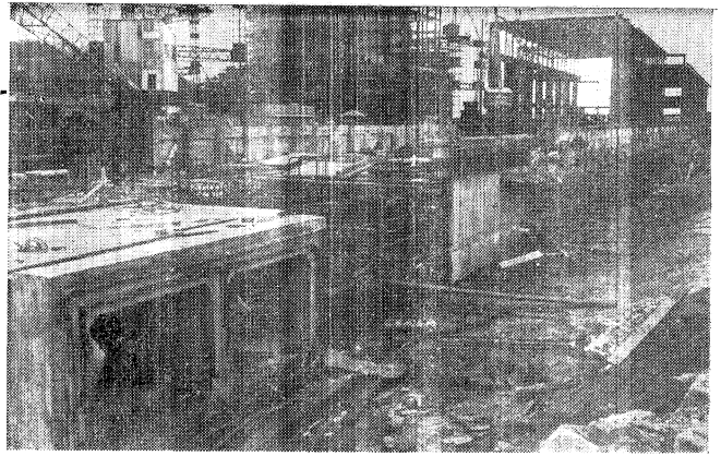
Hunterston 原子力発電所冷却水導水溝ばかりが手前で見える（箱形の）。ゴム製の Water stop が見える。正面は工事中の原子炉建屋の鉄骨建屋の鉄骨、左に起重機の鉄骨が見える。
