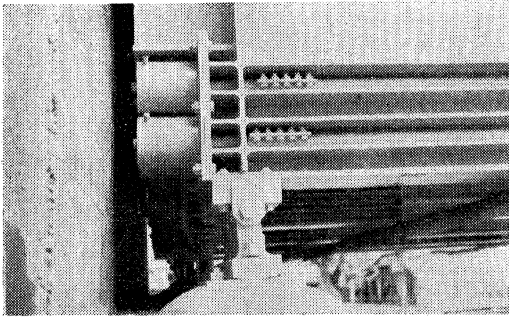
写真-4 新尾形橋の側面（管の中をプレストレス鋼線が通っている）
