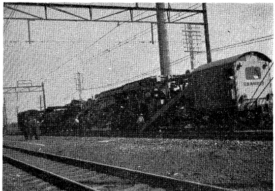
註：右からバラストクリーナ、中間車、ホキ200型ホッパ車（2両）、電源車
