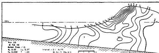
図-3 0.1ftの径の柱にかかる砕波の力の一列 (lb/ft)
